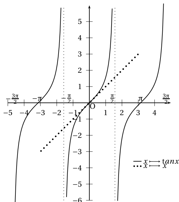
FIGURE 4.7 – Fonction tangente
