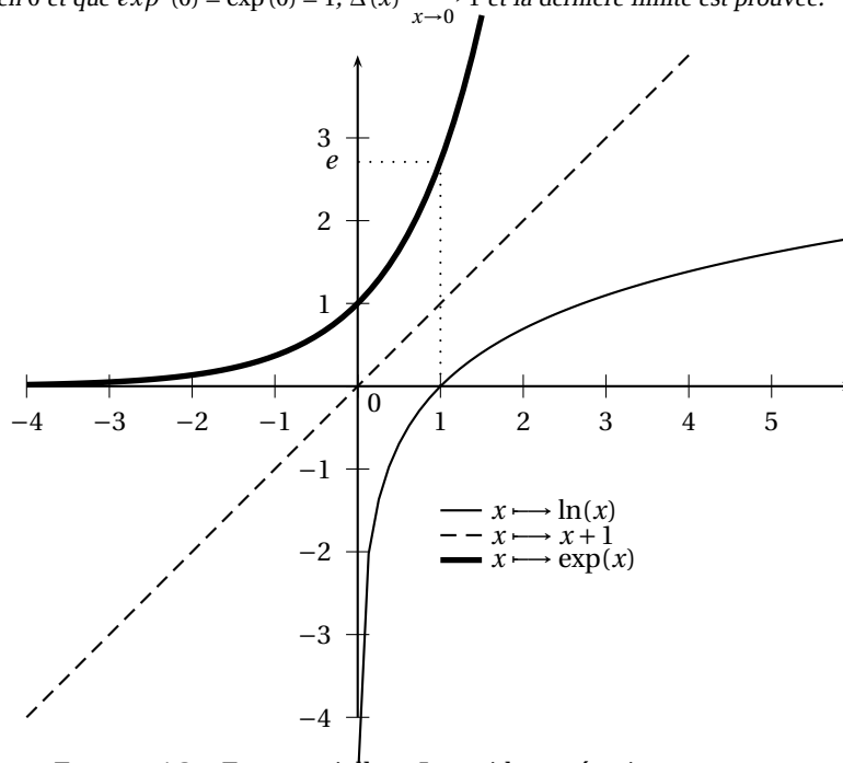
FIGURE 4.2 – Exponentielle et Logarithme népérien
