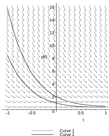
FIGURE 5.1 – Champ de vecteurs et courbes intégrales
