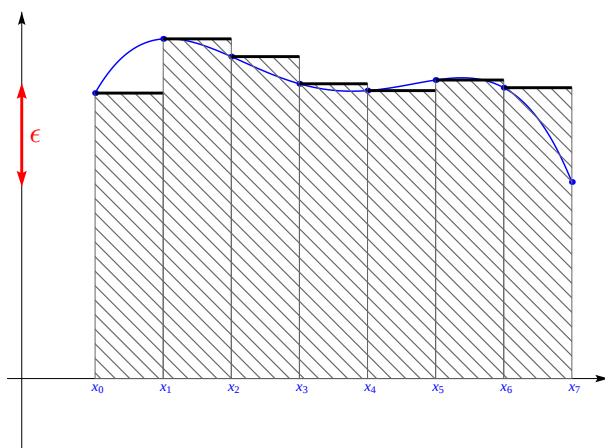
FIGURE 13.7 – Une approximation grossière avec \varepsilon assez grand
