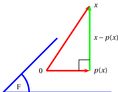
FIGURE 27.2 – Projecteur orthogonal
