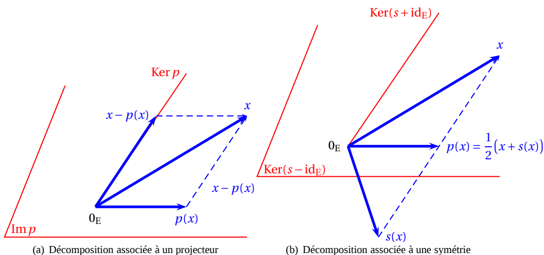
FIGURE 23.5 – Projecteur, symétrie
