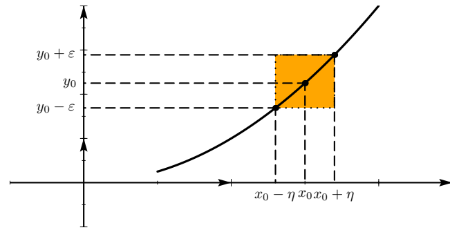
FIGURE 11.2 – Avec \varepsilon = 0.2
