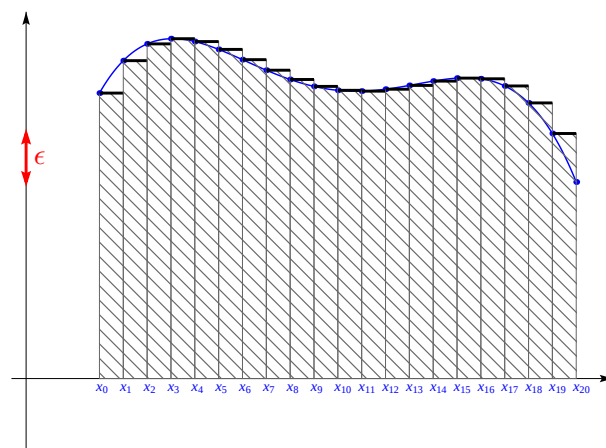
FIGURE 13.8 – Une approximation plus fine avec \varepsilon plus petit
