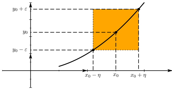
FIGURE 11.1 – Avec \varepsilon = 0.4
