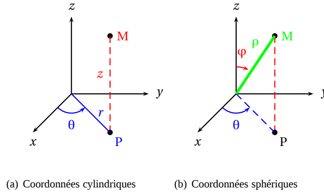
FIGURE 3.3 – Coordonnées cylindriques et sphériques
