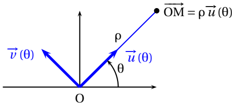
FIGURE 6.4 – Repère polaire : \mathcal{R}_\theta = (O, u(\theta), v(\theta))
