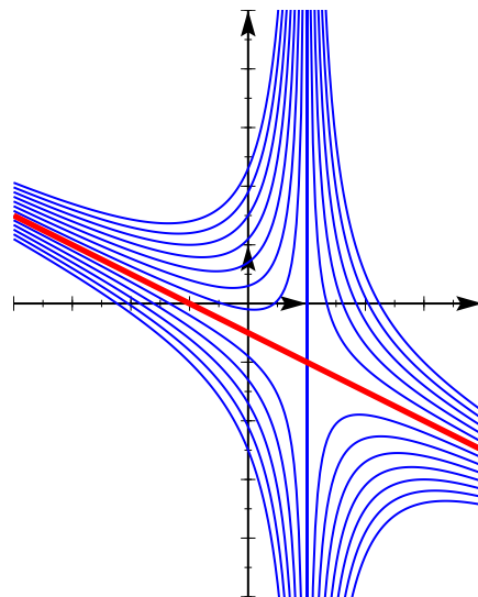
FIGURE 5.4 – Quelques courbes intégrale de (E). On remarquera celle associée à \zeta
