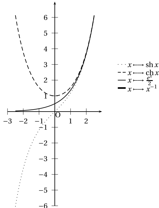
FIGURE 4.12 – Fonctions cosinus et sinus hyperboliques
