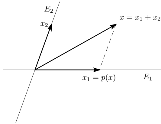
FIGURE 23.3 – Projection sur E_1 parallèlement à E_2
