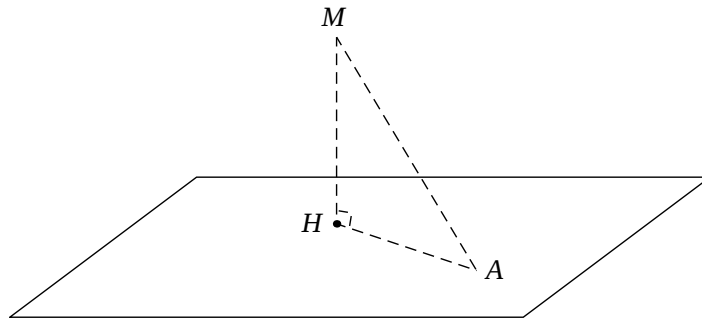
FIGURE 3.7 – Distance d'un point à un plan
