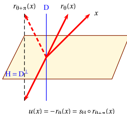
FIGURE 27.6 – Isométrie indirecte avec E(1) = \{0_E\}
